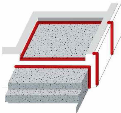
玄関土間打継ぎ部、基礎断熱材接合部の防蟻処理
