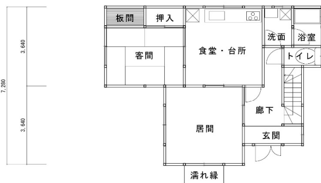
1階平面図 1/100
