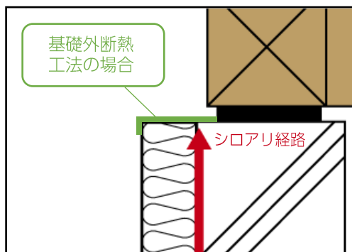
断熱材天端から基礎天端にわたって貼る
